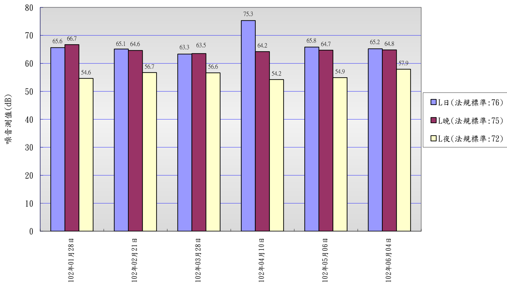
102年01月~06月噪音監測(廠址週界)-第四類管制區之緊鄰8公尺(含)以上之道路
