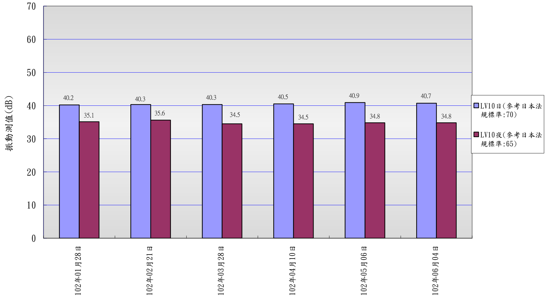
102年01月~06月振動監測(廠址週界)-第二種區域 (法規值係參考日本振動規制法施行細則)
