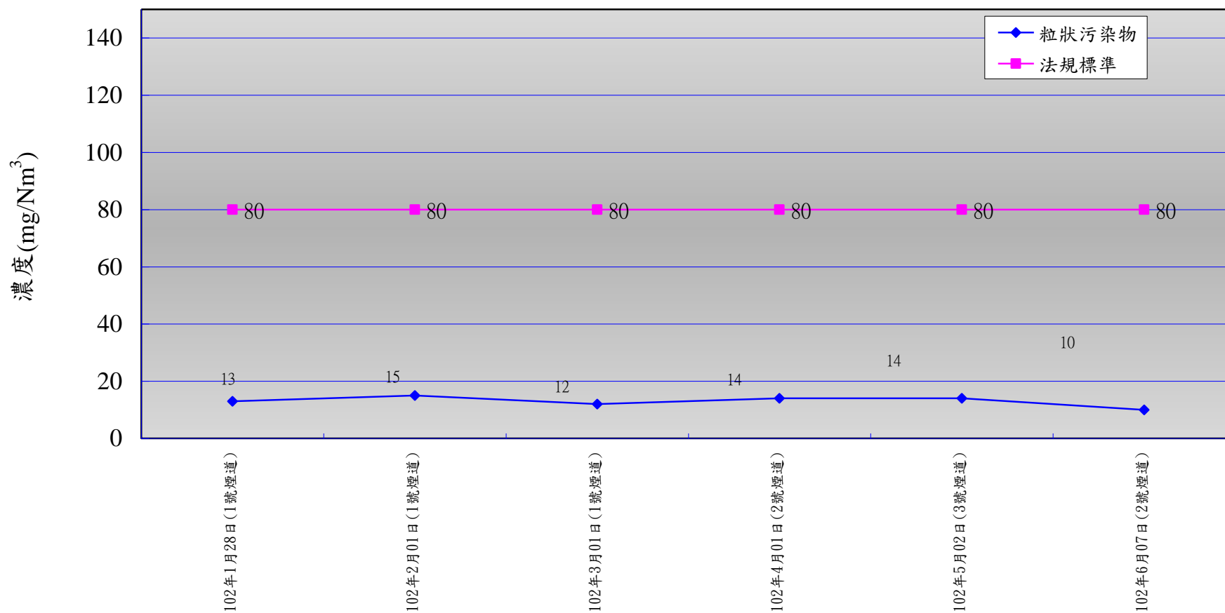
102年01月~06月煙道廢氣檢測結果-粒狀污染物
