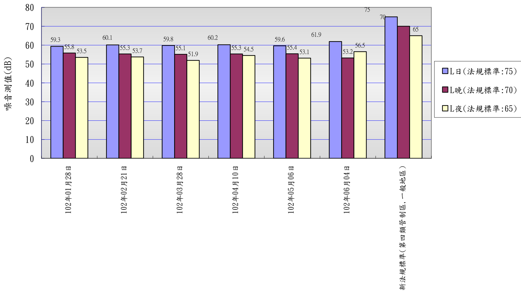
102年01月~06月噪音監測(鼎警新村)-第四類管制區之一般地區
